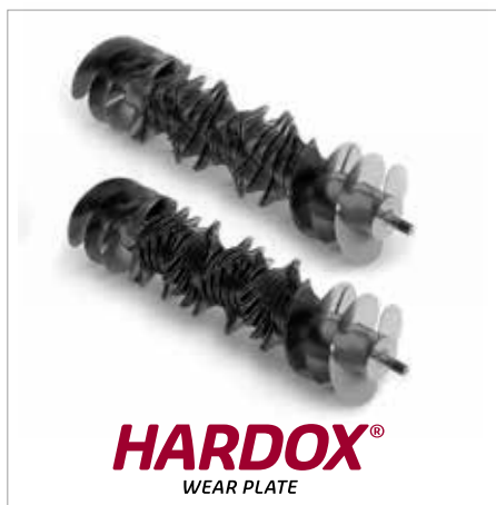
4. ИНТЕГРАЛЬНЫЕ РОТОРЫ с 3 зубьями: / OPTICUT 14 / OPTICUT 23
